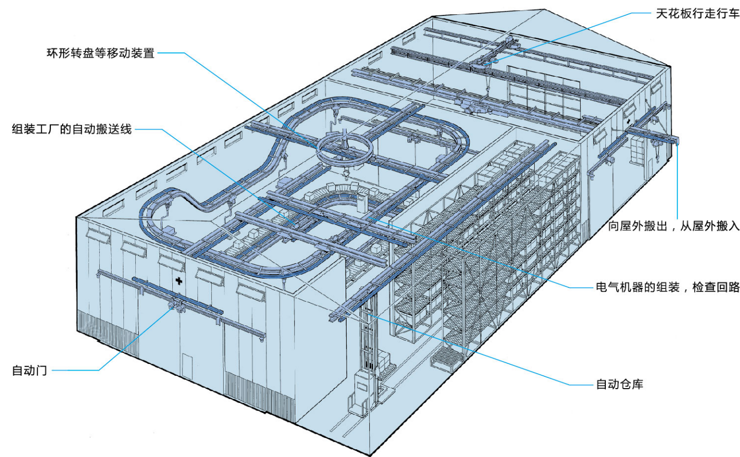
Trolley Duct的系统构成图
