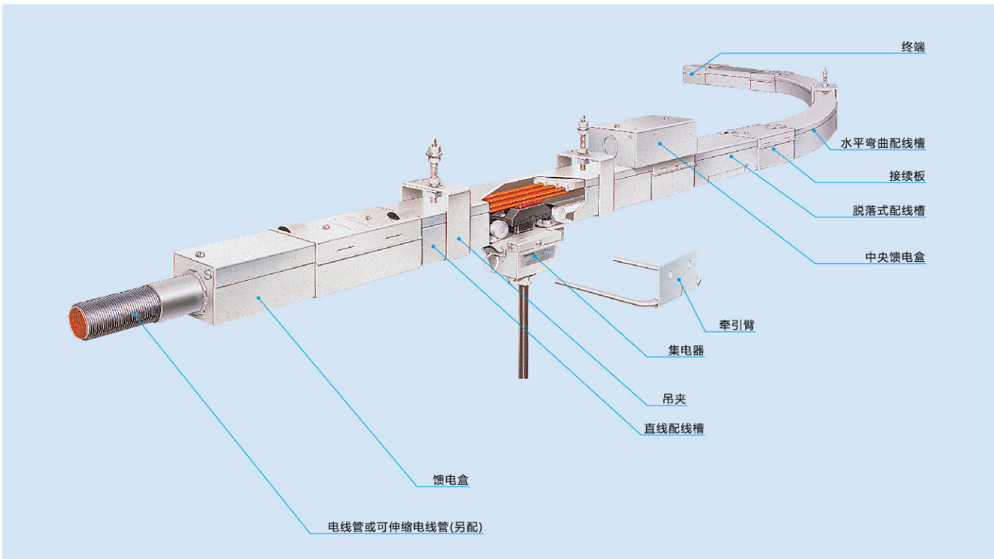
Trolley Duct的系统构成图
