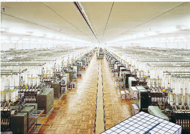
■电动台车
